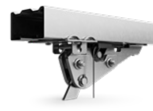
mechanische trolleyvergrendeling
